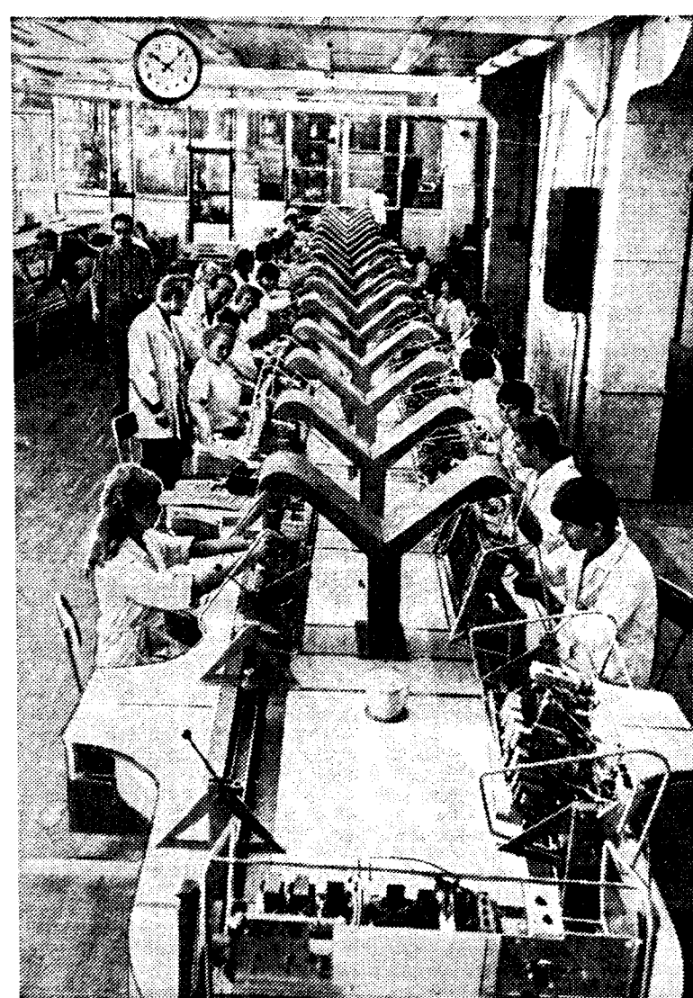
На снимке: конвейер сборки радиола «Эстония-стерео». Фото ТАСС.
